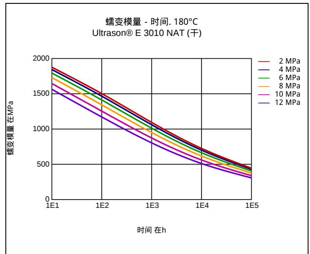
蠕变模量 - 时间. 180°C
